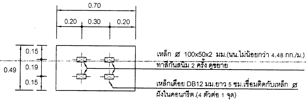
แปลนฝาบ่อพัก ไม่ได้มาตราส่วน
