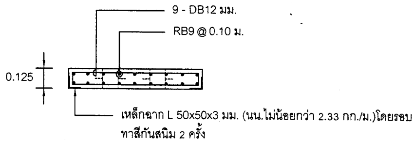
รูปตัดฝาบ่อพัก ไม่ได้มาตราส่วน
