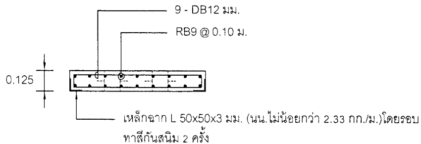
รูปตัดฝ่าวบ่อกัก ไม่ได้มาตรฐาน
